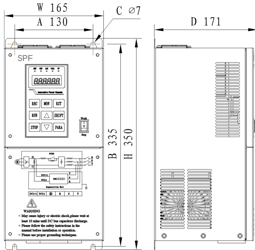
图 3-1 C1 壁挂式机箱外形尺寸和安装尺寸
