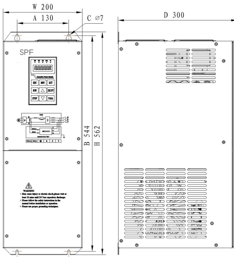
图 3-3 C3 壁挂式机箱外形尺寸和安装尺寸
