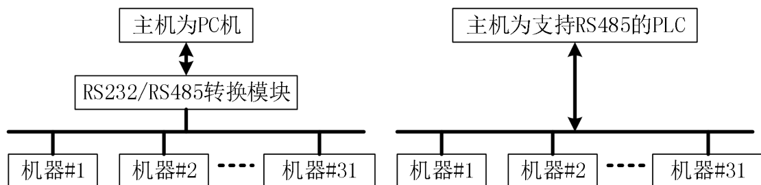
图 5-2 单主机多从机组网方式示意图
