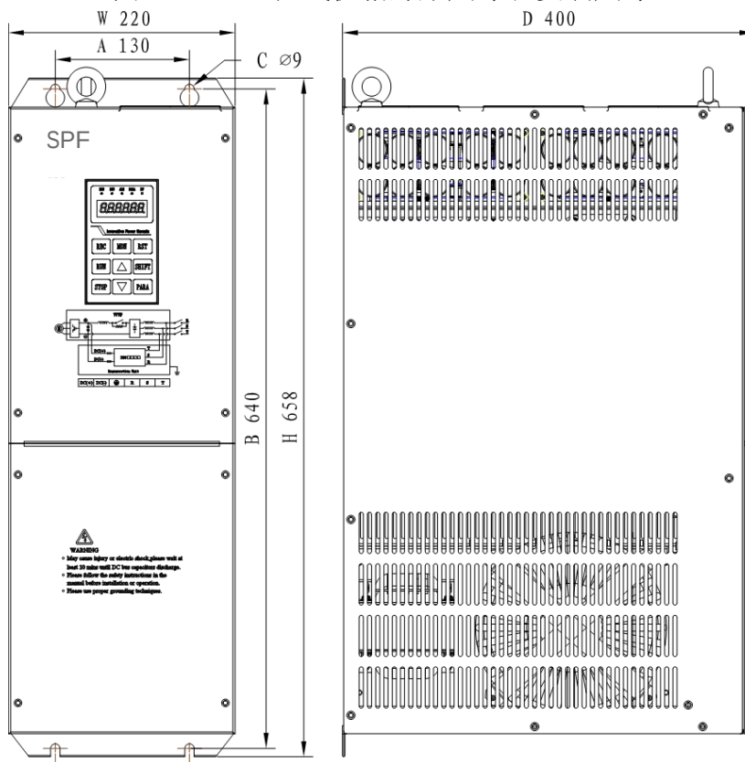
图 3-4 C4 壁挂式机箱外形尺寸和安装尺寸
