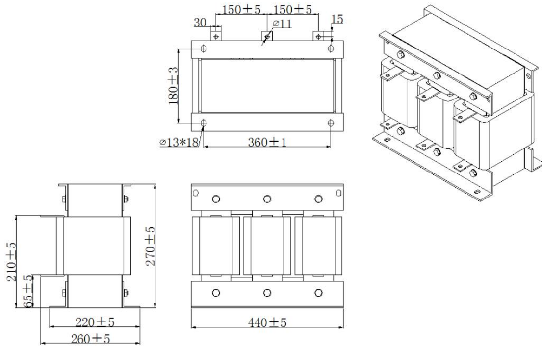
图 3-7 外置电抗器 SPF-PF-150/0.5-L 外形尺寸和安装尺寸
