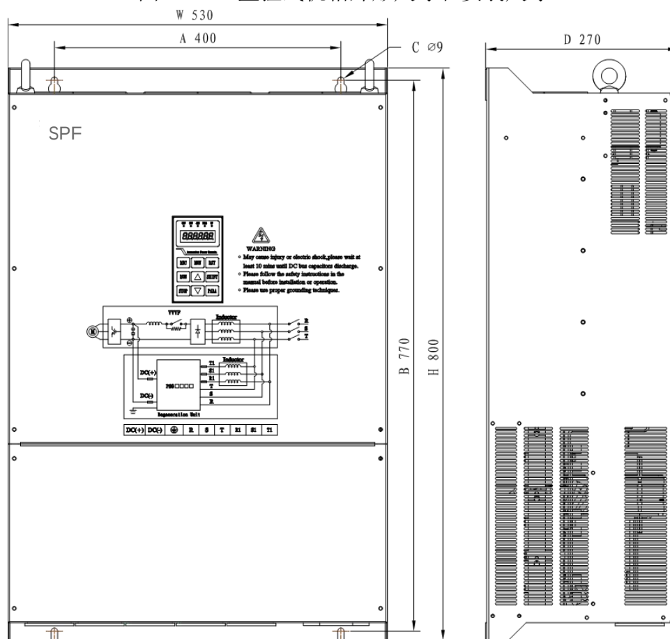
图 3-6 C6 壁挂式机箱外形尺寸和安装尺寸
