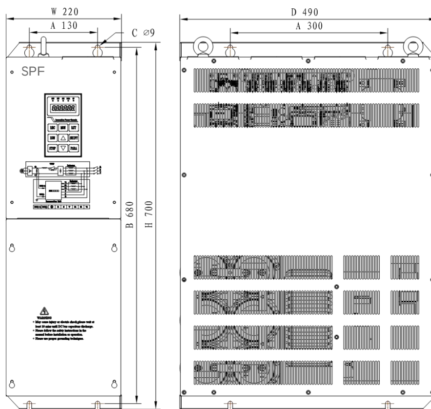
图 3-5 C5 壁挂式机箱外形尺寸和安装尺寸
