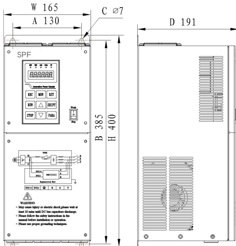
图 3-2 C2 壁挂式机箱外形尺寸和安装尺寸
